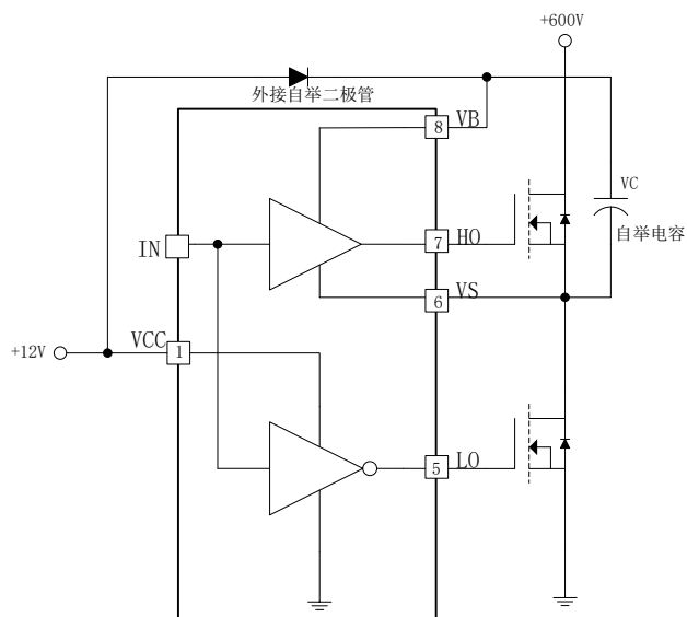
图 8-3. EG2104S 自举电路结构
